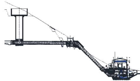
HES No:3 - Cebri Boru HES No:3 - Penstock
